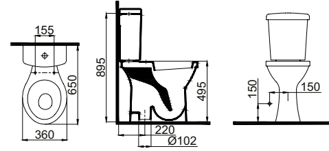
2204-0105 Bedensel Engelli Alttan Çıkışlı Klozet (36x65x49) S-Trap WC Pan
